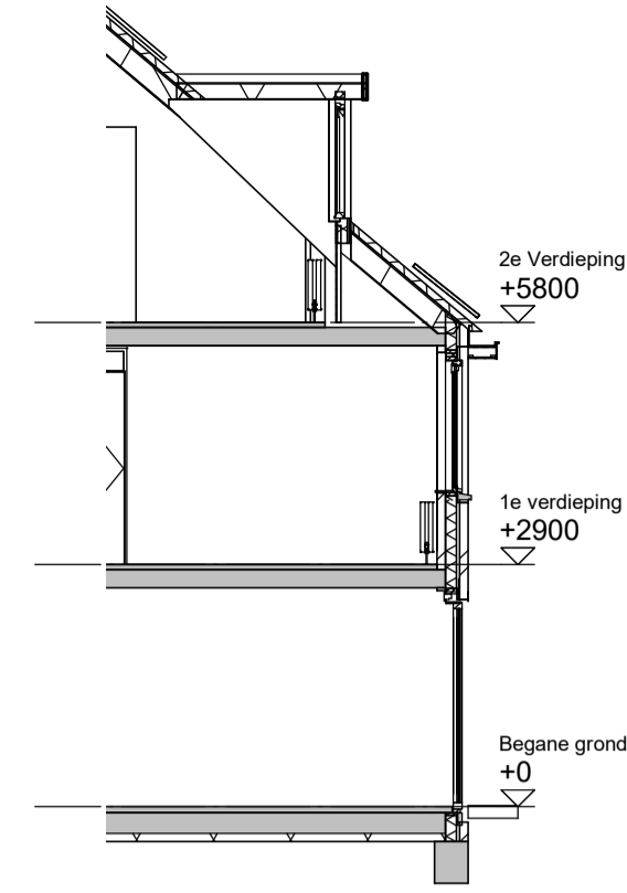
Doorsnede A1-O3 -optie dakkapel achtergevel (vergunningsvrij)
