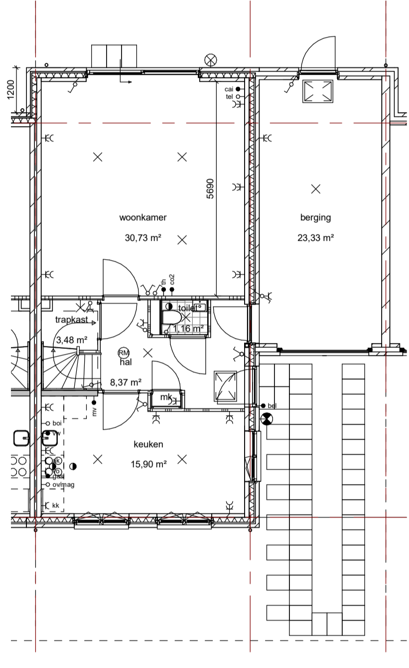
Begane grond -optie uitbouw achtergevel 1,2m (vergunningsvrij)
