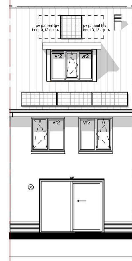
Achtergevel -optie dakkapel achtergevel (vergunningsvrij)
