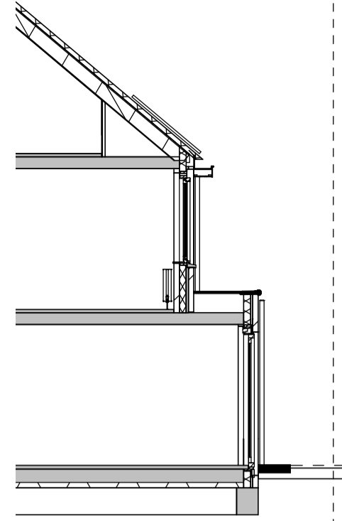
Doorsnede -optie uitbouw achtergevel 1,2m (vergunningsvrij)
