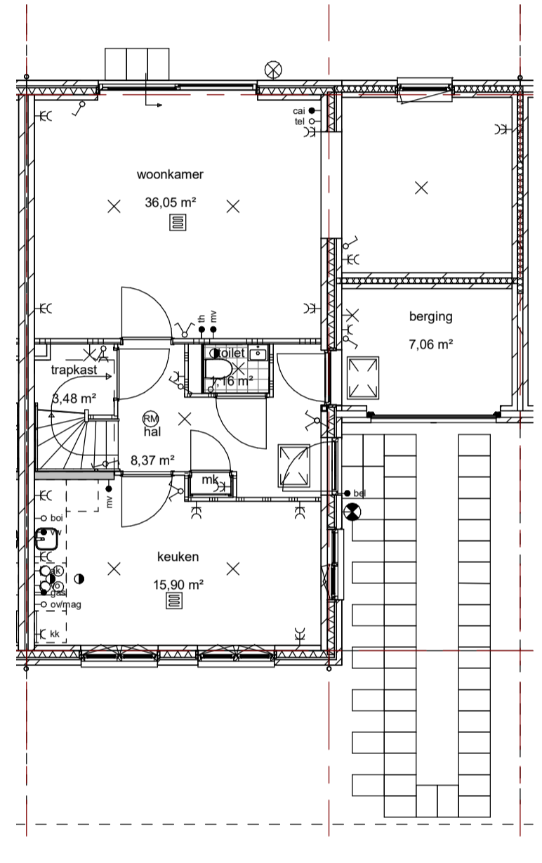
Begane grond -optie uitbreiding woonkamer - glaskozijn met ventilatie rooster (vergunningsvrij)
