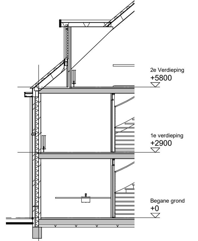
Doorsnede A1-O4 -optie dakkapel voorgevel (vergunningplichtig) bij deze optie komt er een extra pv-paneel bij bnr 9.10 en 13
