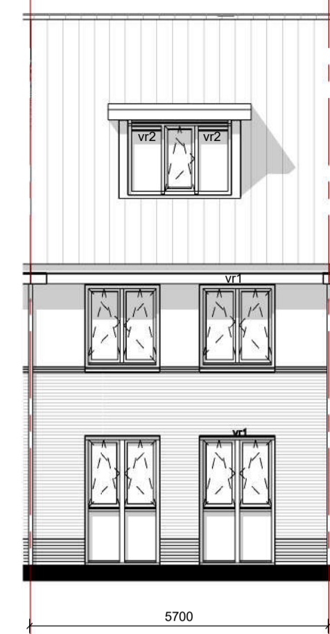
Voorgevel -optie dakkapel voorgevel (vergunningplichtig) bij deze optie komt er een extra pv-paneel bij bnr 9.10 en 13
