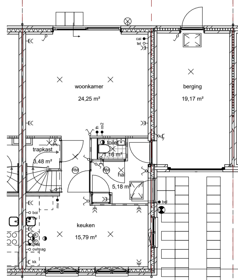
Begane grond -optie uitbreiding woonkamer - glaskozijn met ventilatie rooster (vergunningsvrij)
