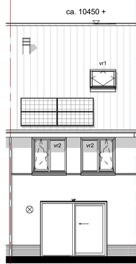
Achtergevel -optie dakraam achtergevel (vergunningsvrij)
