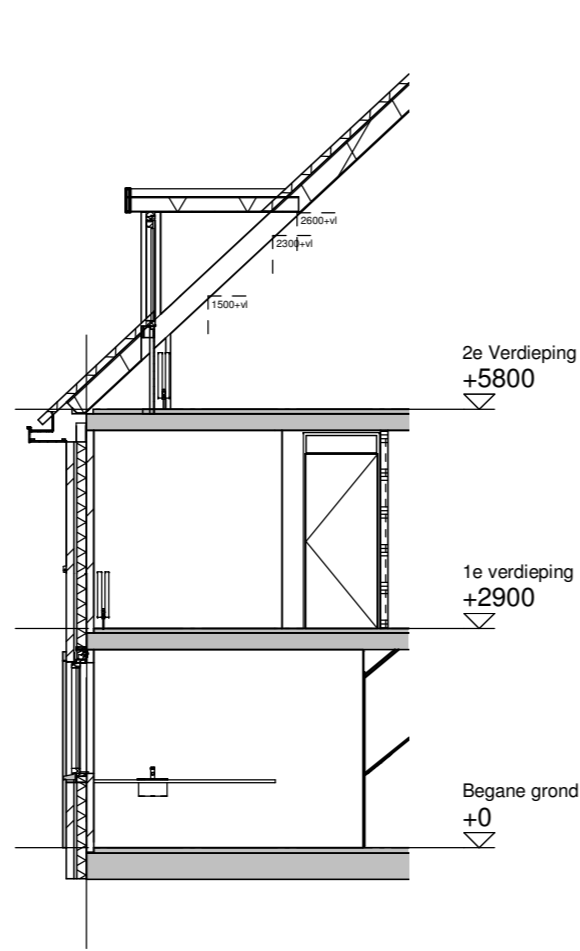
Doorsnede A1-O4 -optie dakkapel voorgevel (vergunningplichtig)
