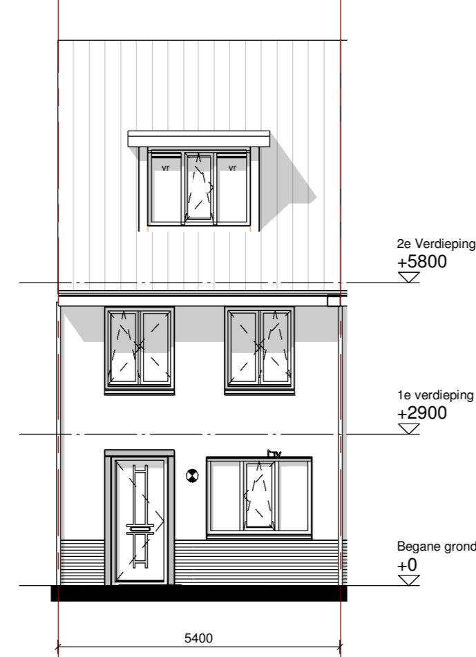
Voorgevel -optie dakkapel voorgevel (vergunningplichtig)
