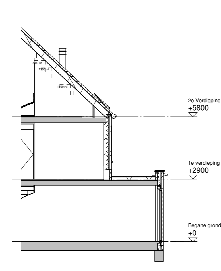
Doorsnede A1-O5 -optie uitbouw 1,2m achtergevel (vergunningsvrij)
