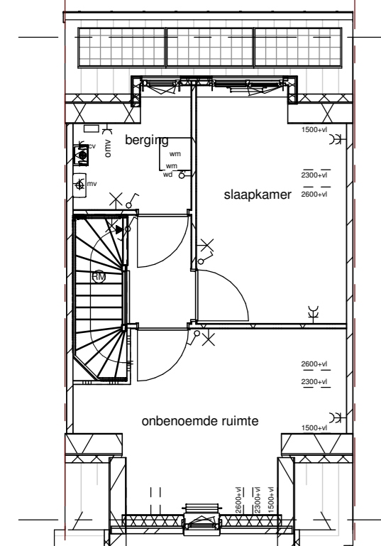
2e verdieping (tuitgevel) -dakkapel achtergevel (vergunningsvrij) -optie zolderindeling (vergunningsvrij)
