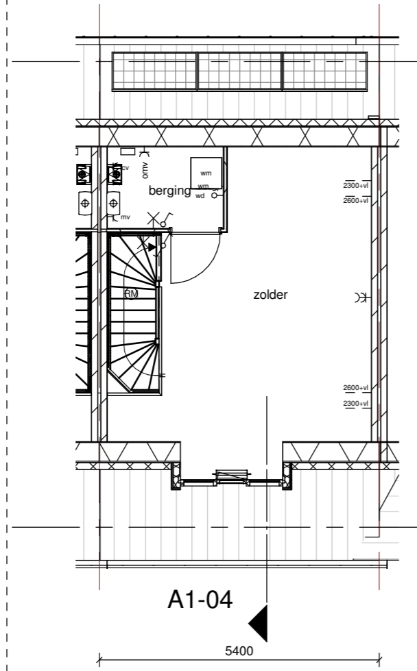
2e verdieping -optie dakkapel voorgevel (vergunningplichtig)
