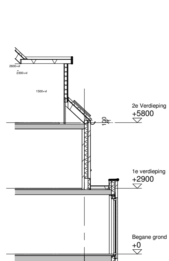
Doorsnede A1-O3 -optie dakkapel achtergevel (vergunningsvrij) (alleen mogelijk bij hofwoningen)
