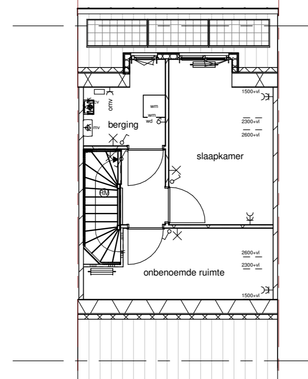
2e verdieping -dakkapel achtergevel (vergunningsvrij) -optie zolderindeling (vergunningsvrij)
