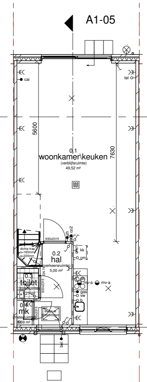
Begane grond -optie uitbouw 1,2m achtergevel (vergunningsvrij)
